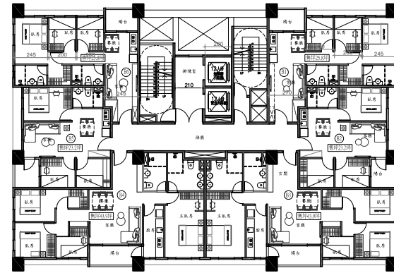
B棟 3F-22F S:1/100
