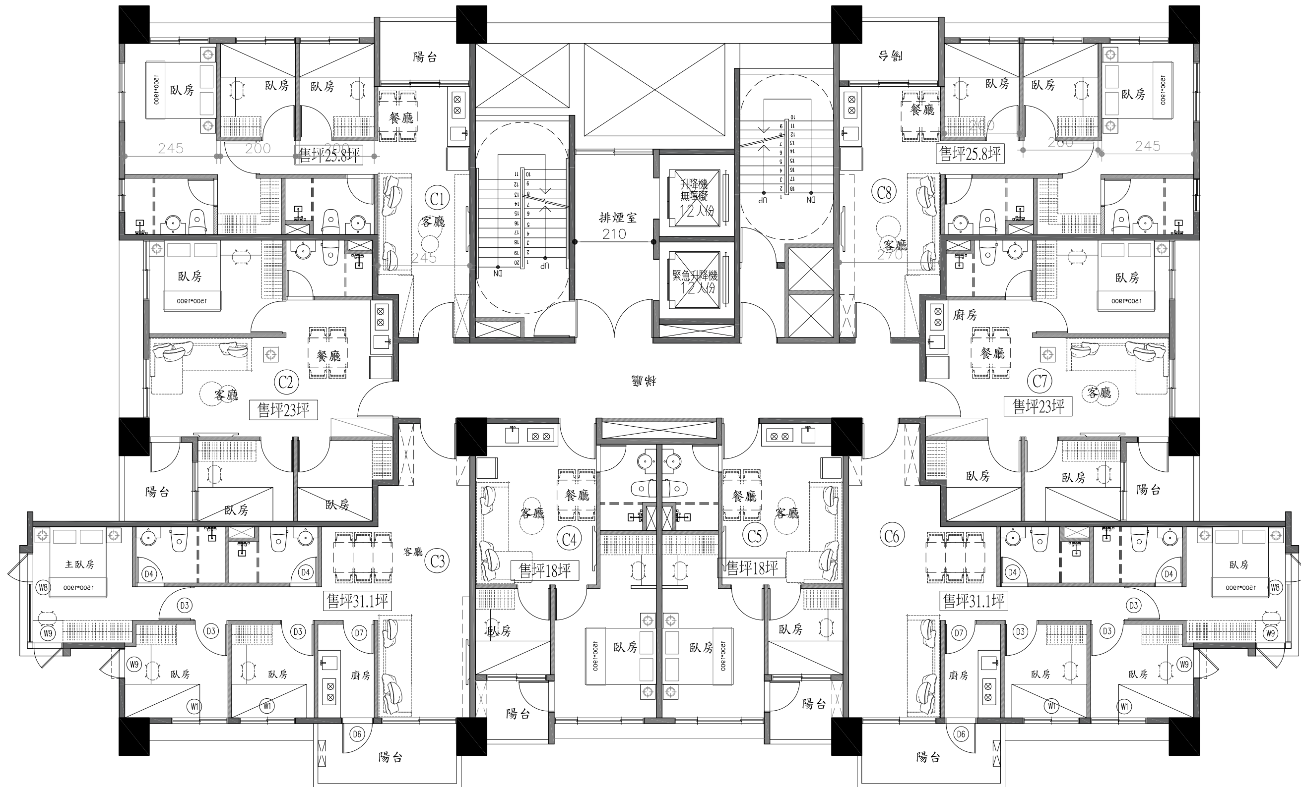
C棟 3F-21F S:1/100
