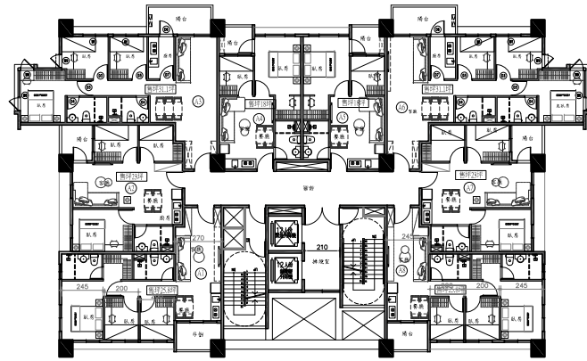
A棟 3F-21F S:1/100
